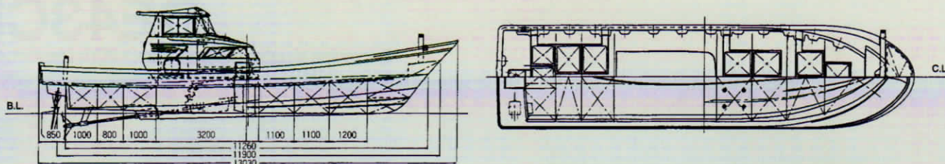
○一般配置図(単位:mm)
