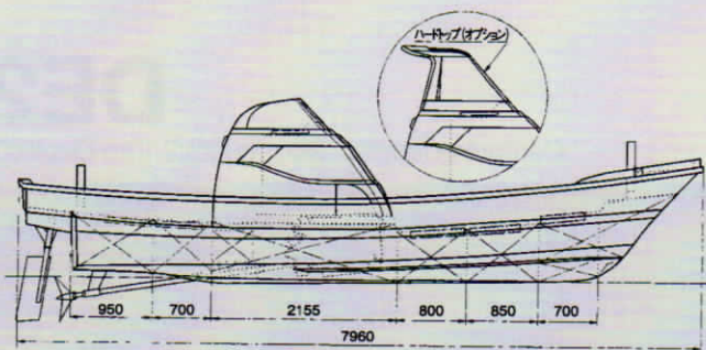
○一般配置図(単位:mm)
