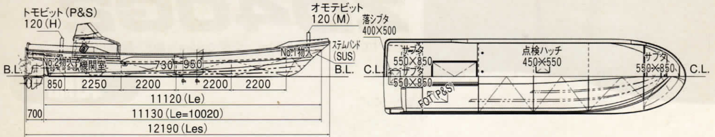
■一般配置図(単位:mm)
