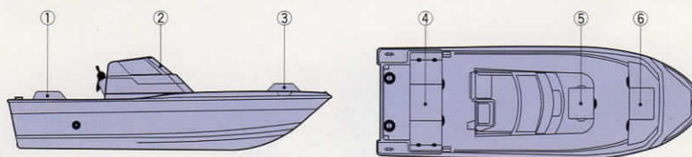
①スターンレール ②ウインドシールド ③パウレール ④スタンロッカー ⑤イケス ⑥アンカーストア
